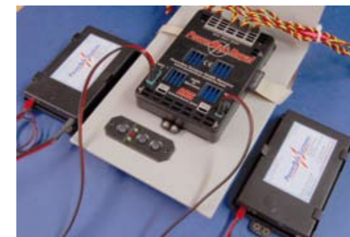
Zwei PowerBox-Akkus mit 2.800 Milliamperestunden Kapazität versorgen die PowerBox Royal
