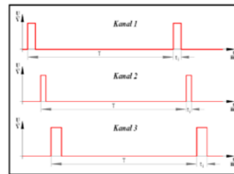
Abb. 1: Parallele Servo-Impulsausgabe
