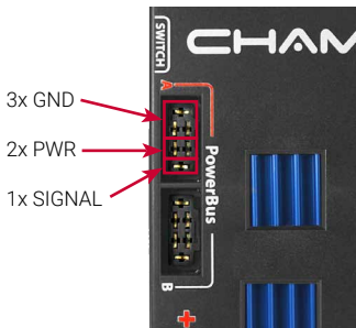
PowerBUS Buchse
